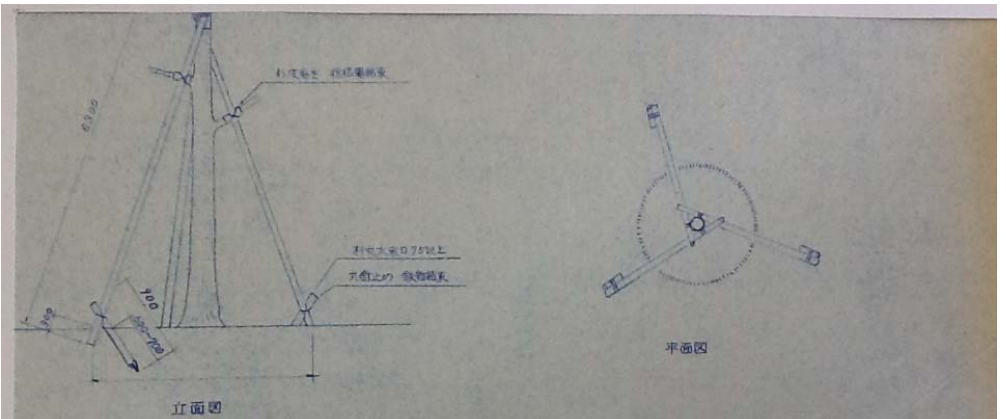
三脚長丸木支柱
