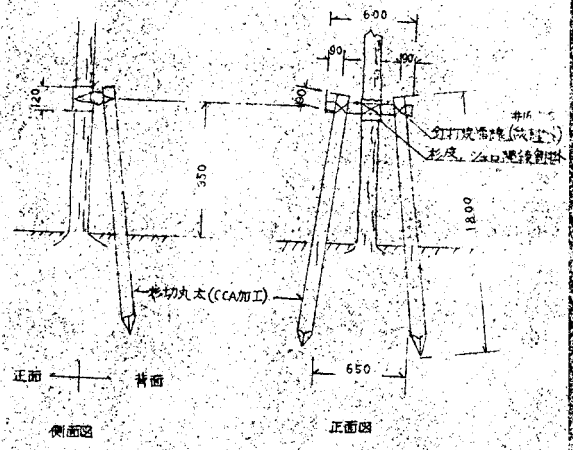
二脚馬居
