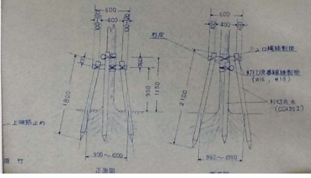
十字鳥居
