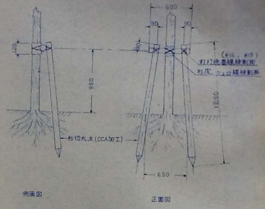
二脚鳥居
