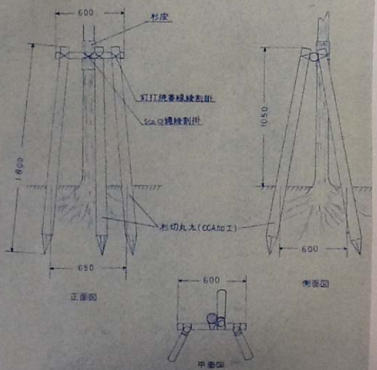
三脚鳥居
