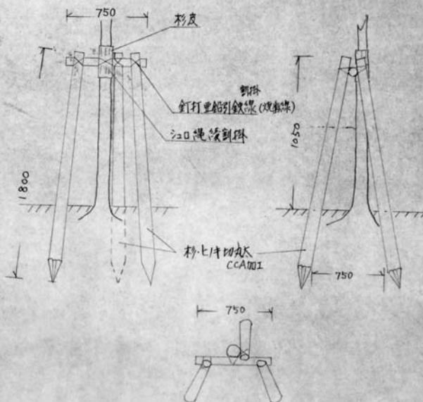
三脚鳥居
