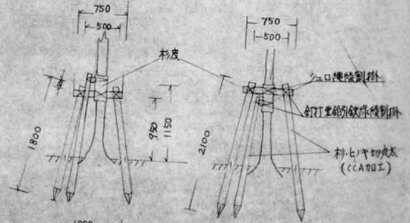
十字鳥居
