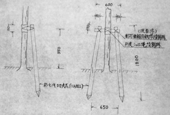
二脚鳥居
